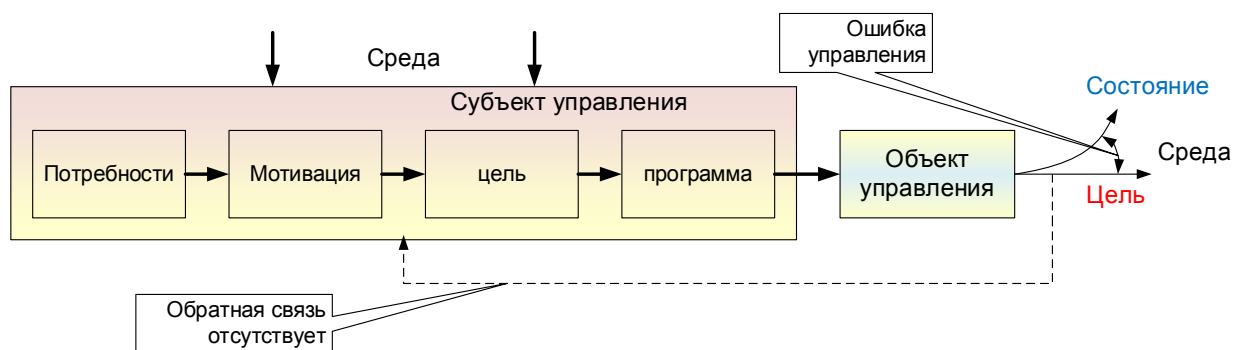
Рисунок 2 – Метод «править»
