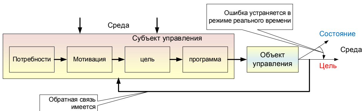
Рисунок 3 – Метод «регулирование»
