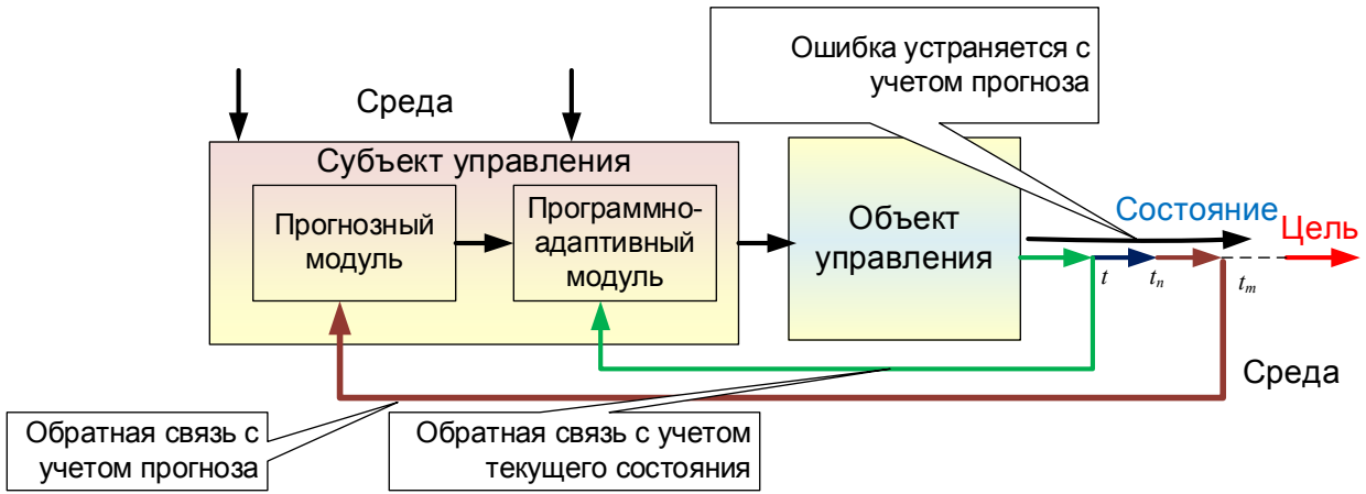
Рисунок 4 – Метод «управление»
